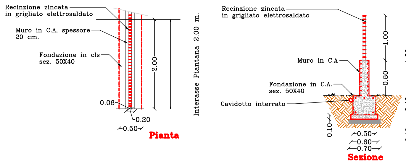
Pianta sezione e prospetto tipo recinzione scala 1:50
